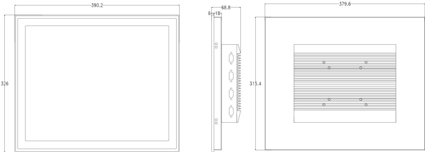
嵌入尺寸：379.6*315.4 面板尺寸：390.2*326 壁挂尺寸：100*100 75*75
